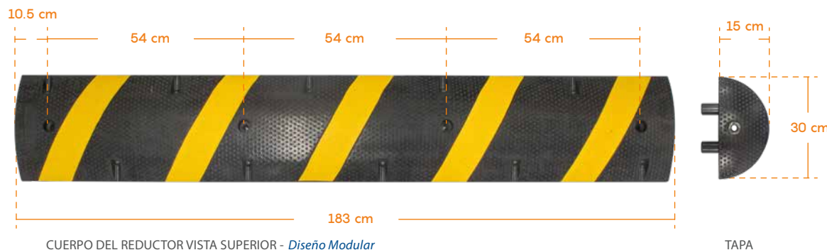
CUERPO DEL REDUCTOR VISTA SUPERIOR - Diseño Modular
